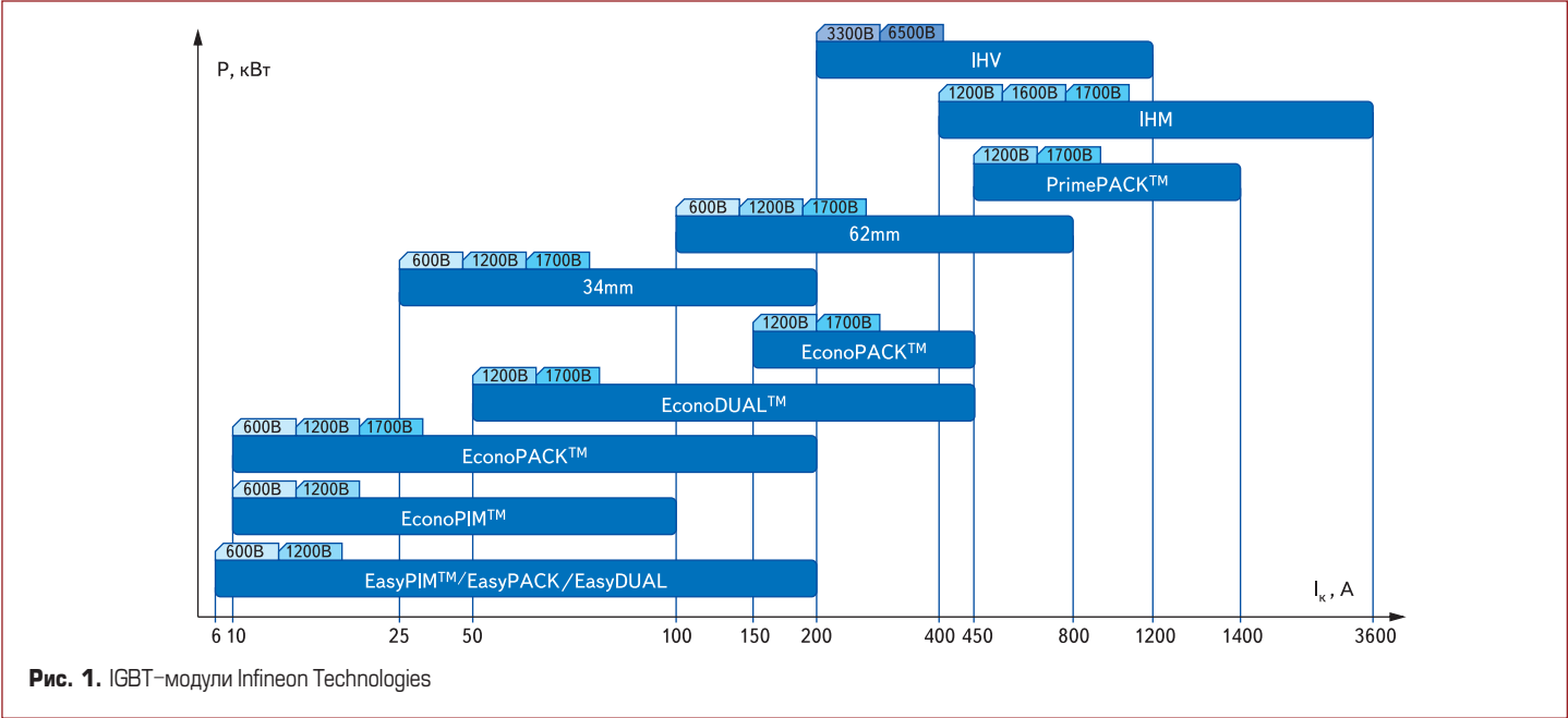
Рис. 1. IGBT-модули Infineon Technologies
